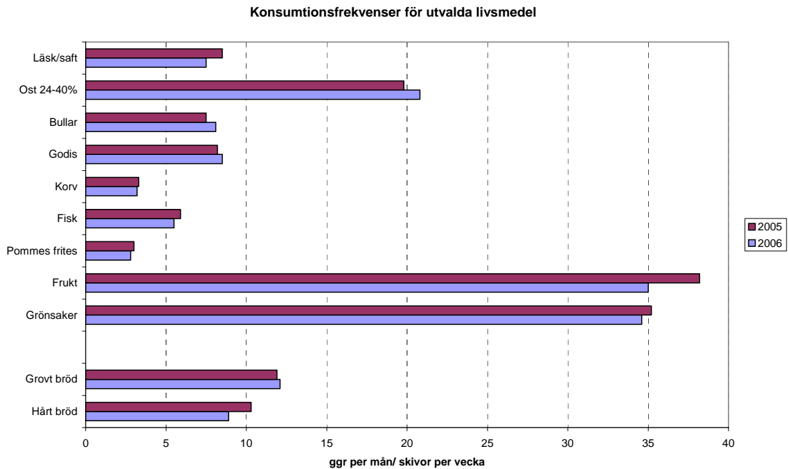
Figur 2. Konsumtionsfrekvenser för utvalda livsmedel 2005 och 2006
